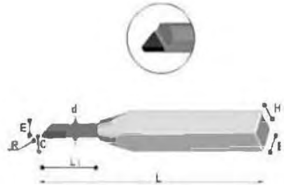
Freze Bıçağı
